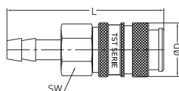
Panel Mount Standard Hose Barb Coupling Kupplung mit Schottverschraubung Schlauchanschluss
