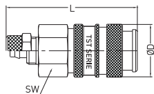
Plastic Hose Coupling Kupplung für Kunststoffschlauch
