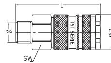
Male Threaded Coupling Kupplung mit Aussengewinde
