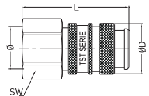
Female Thread Coupling Kupplung mit Innengewinde
