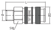
Male Thread Coupling Kupplung mit Aussengewinde
