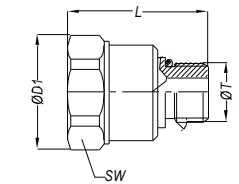
Male Thread Coupler (ISO 6149-2) Kupplung mit Aussengewinde (ISO 6149-2)
