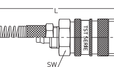
Plastic Hose Coupling With Spring Kupplung für Kunststoffschlauch mit Knickschutzfeder
