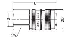
Female Thread Coupling Kupplung mit Innengewinde
