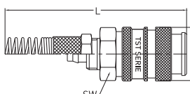
Plastic Hose Couplings With Spring Kupplung für Kunststoffschlauch mit Knickschutzfeder
