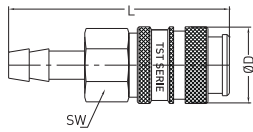
Standard Hose Barb Coupling Kupplung mit Schlauchülse
