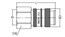
Female thread Coupling Kupplung mit Innengewinde
