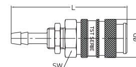
Panel Mount Standard Hose Coupling Kupplung mit Schottverschraubung Schlauchanschluss
