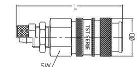
Panel Mount Plastic Hose Coupling Kupplungen mit Schottverschraubung für Kunststoffschlauch
