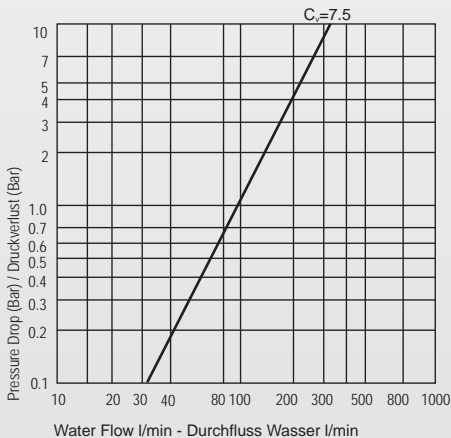
Hose Tail Shut-Off Plug Nippel Mit Schlauchtülle -absperrend
